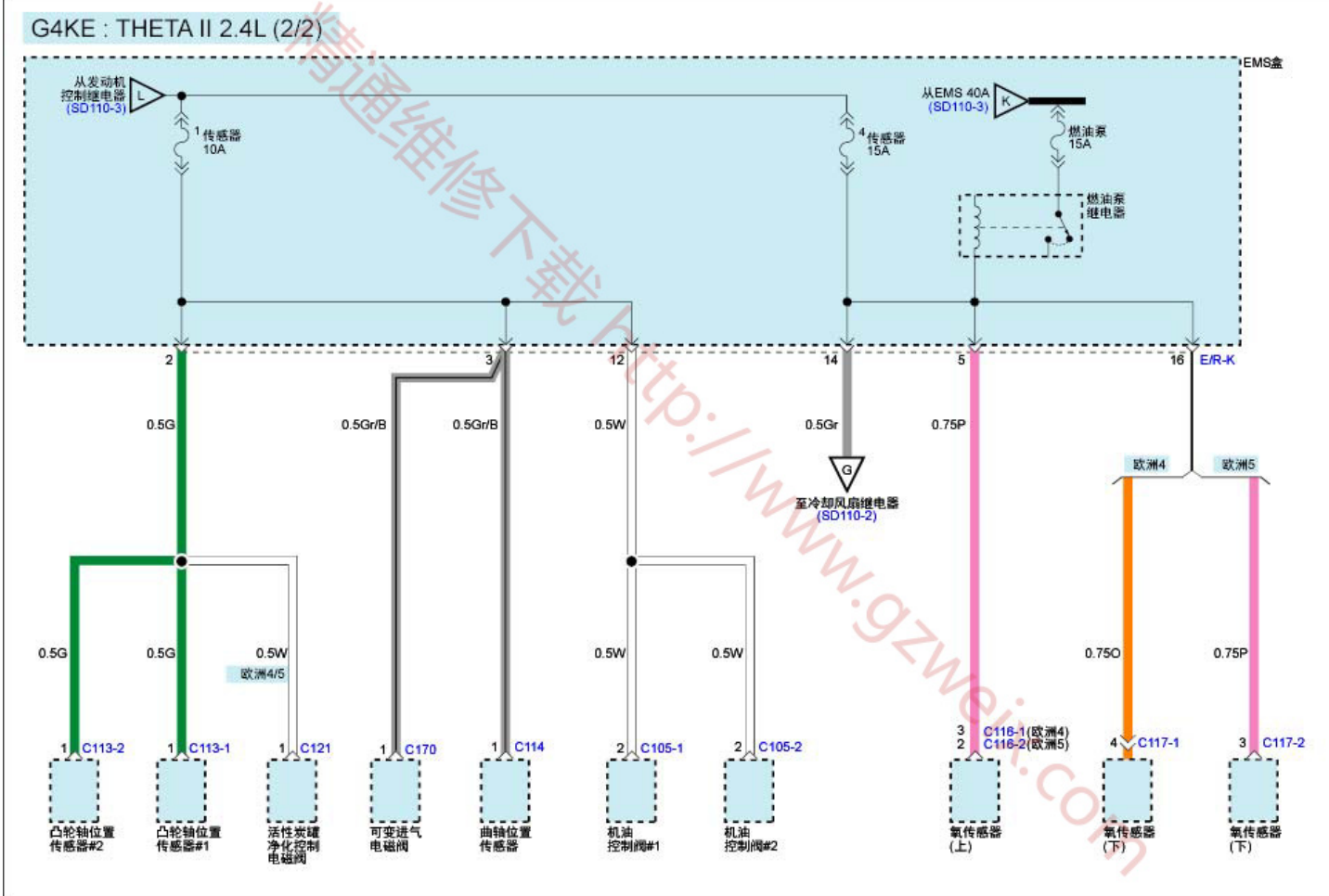
电源分布(4)
